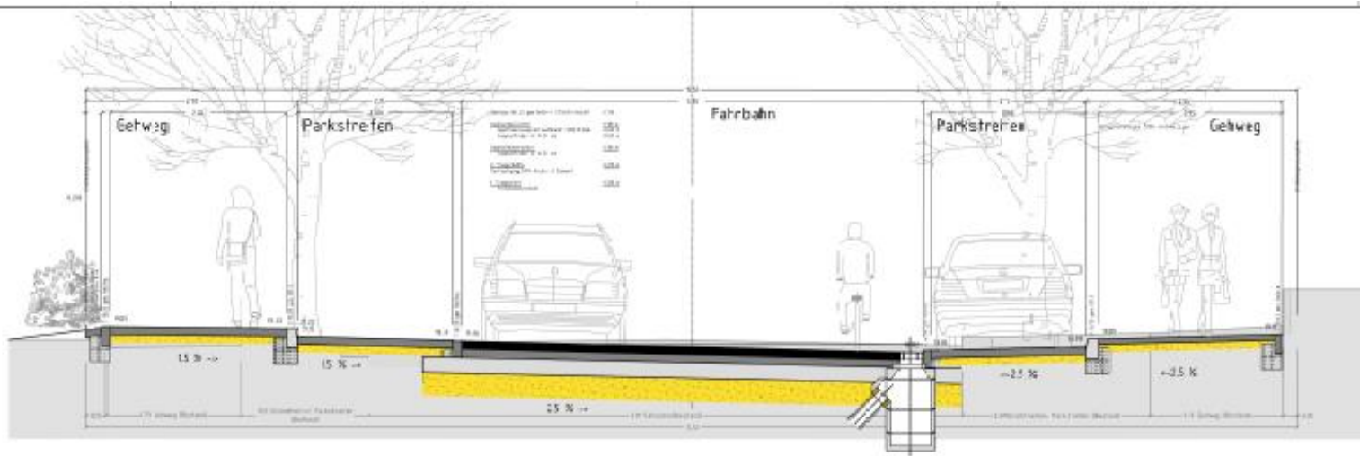
Schnitt M 1:25
